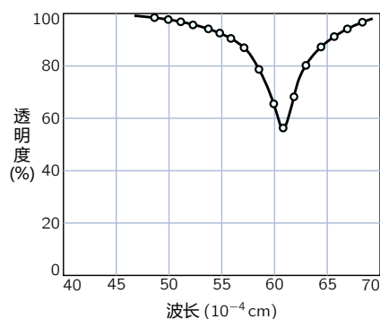
图 23.6: 通过一个薄氯化钠膜 ( 0.17 \mu m ) 的红外辐射透射
