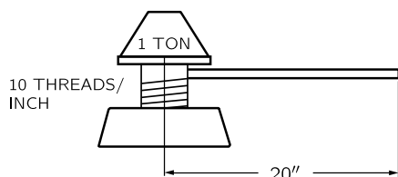
图 4.5: 螺旋起重器
